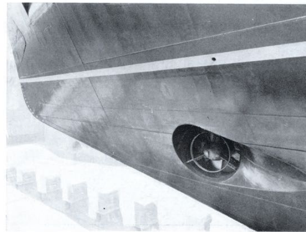
OHJAUSPOTKURI KEULALAIVASSA STYRPROPELLERN I FÖRSKEPPET STEERING PROPELLER IN THE BOW
